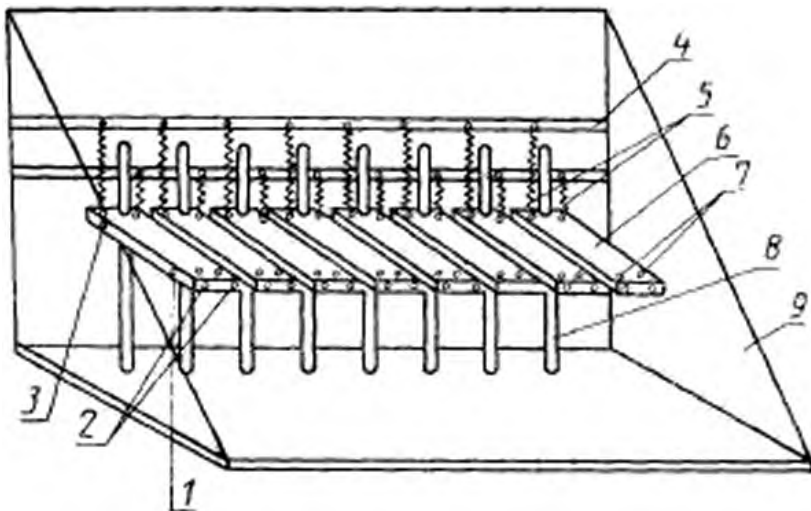
1 — мульти-канал электродов; 2 — токковод; 3 — винт-фиксатор держателя; 4 — винт-пробка; 5 — гибкий провод; 6 — держатель; 7 — отверстие для электрода; 8 — стойка; 9 — корпус из оргстекла
