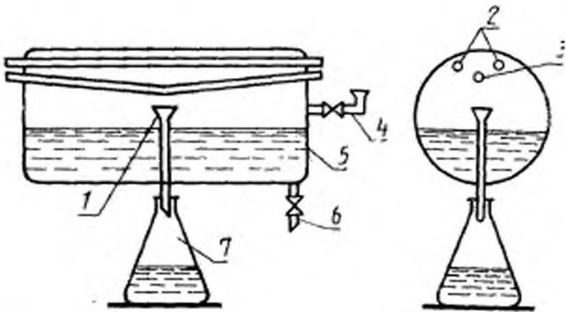
1 — воронка; 2 — нагреватель; 3 — холодильник; 4 — край для залива кислоты; 5 — колба; 6 — край для слива кислоты; 7 — колба
